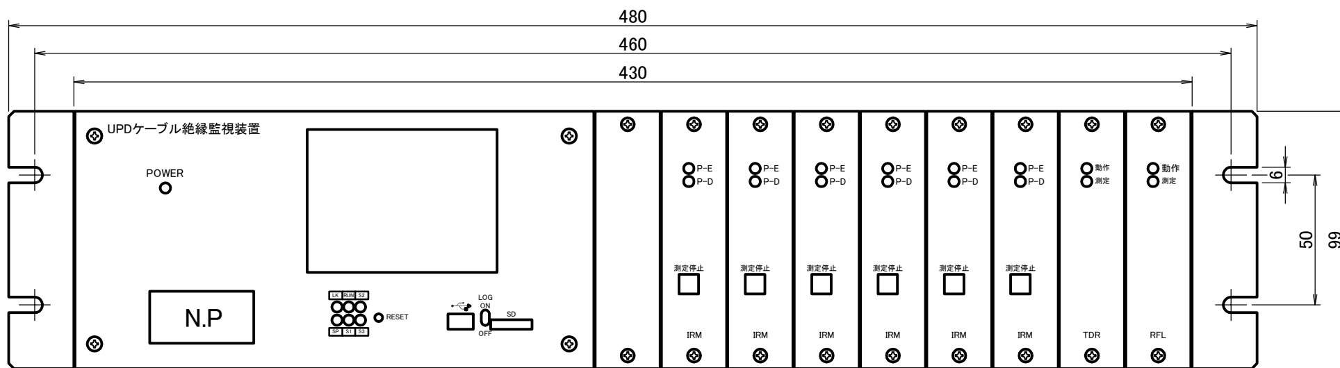
正面図
