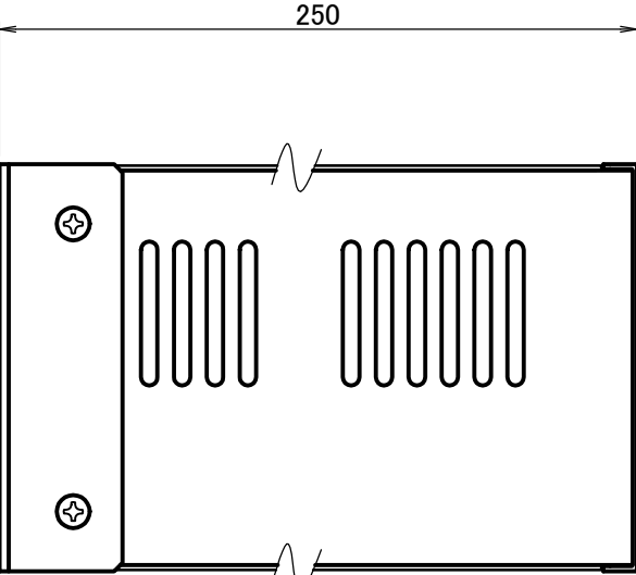
側面図
