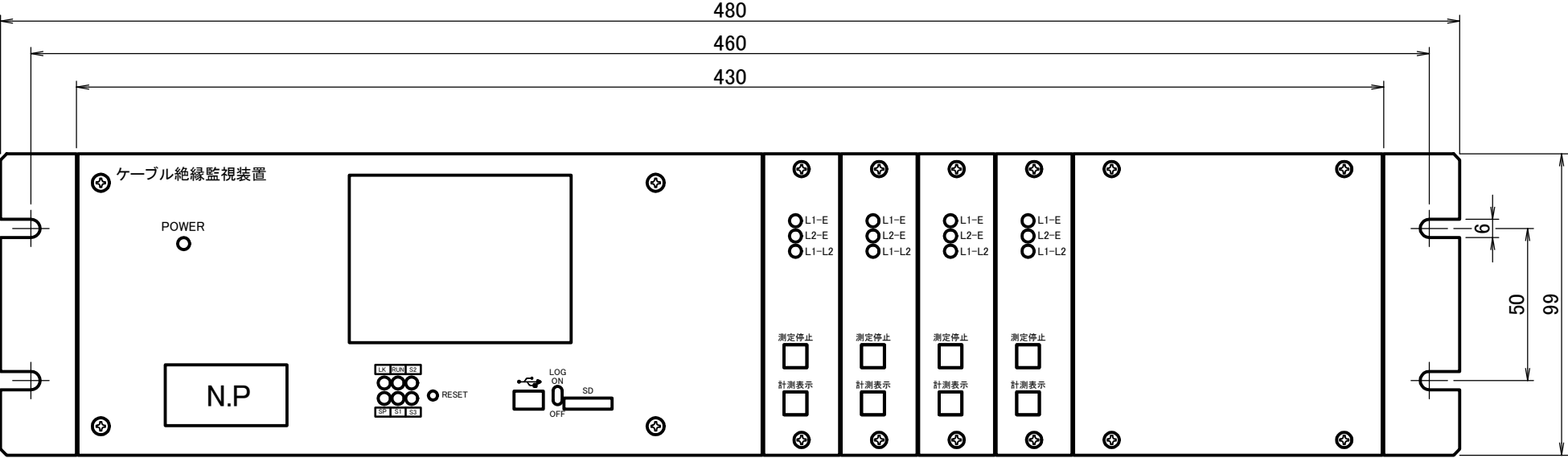
正面図
