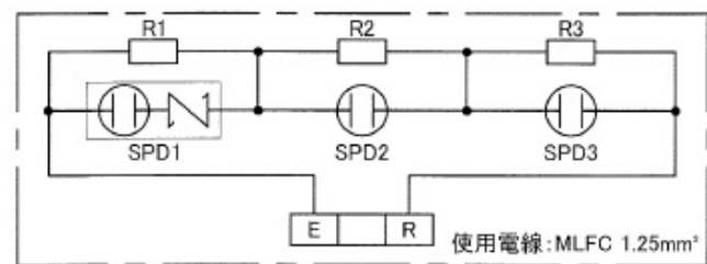
回路図
