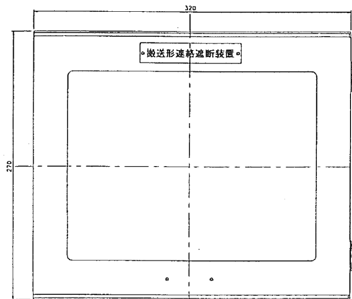
《正面図》
