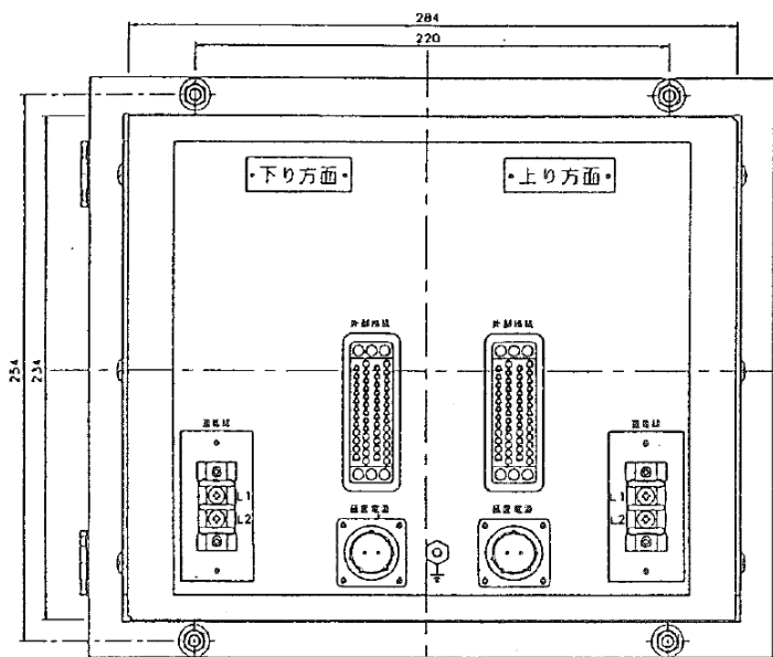
《背面図》
