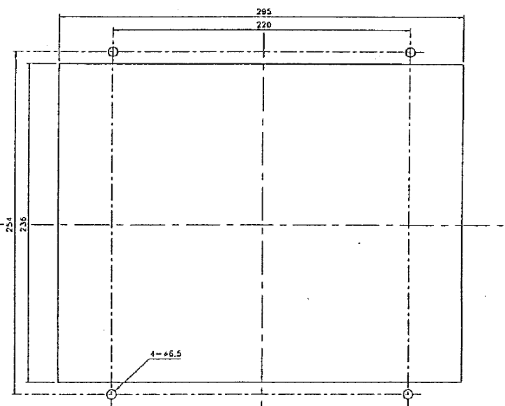
《盤取付穴寸法図》
