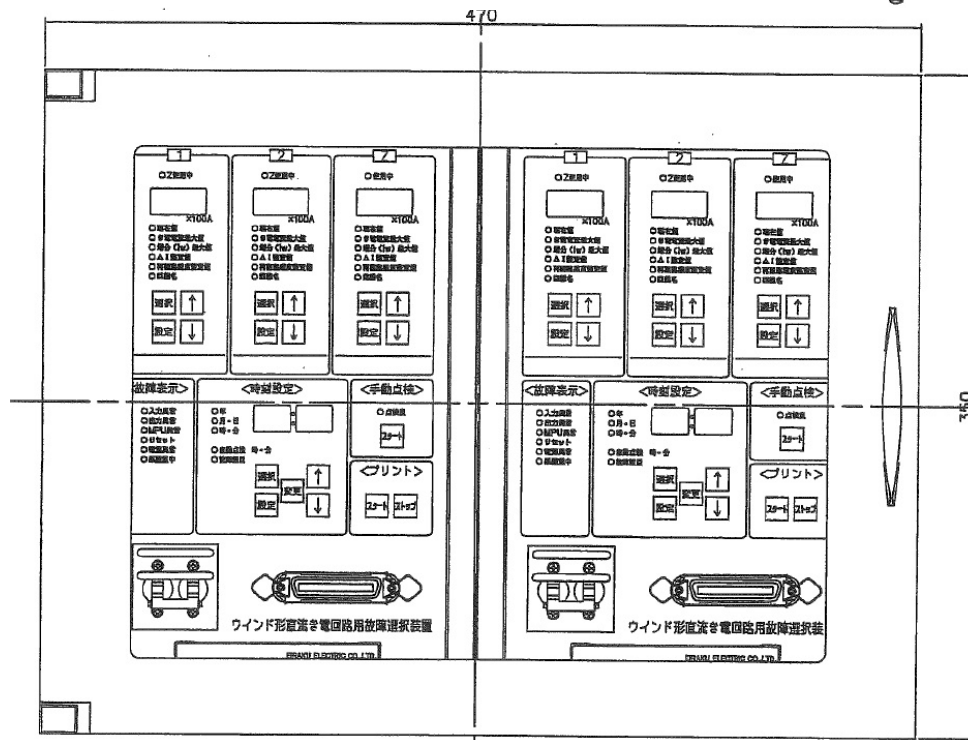
正面図
