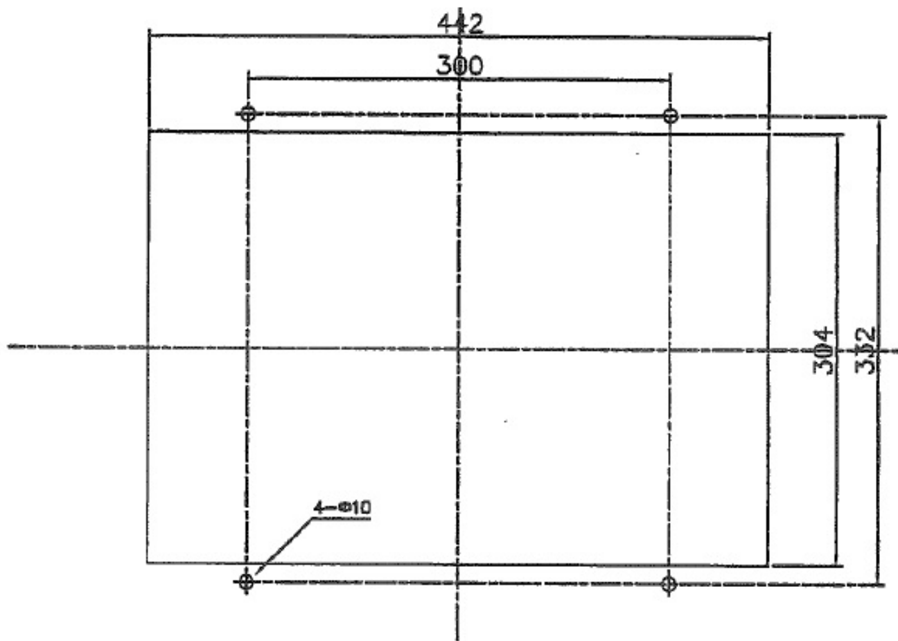
パネルカット図
