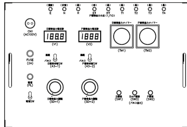
EGG-T 外観図
