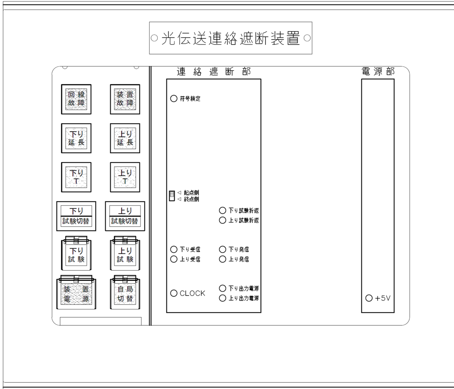
前面パネル実装図
