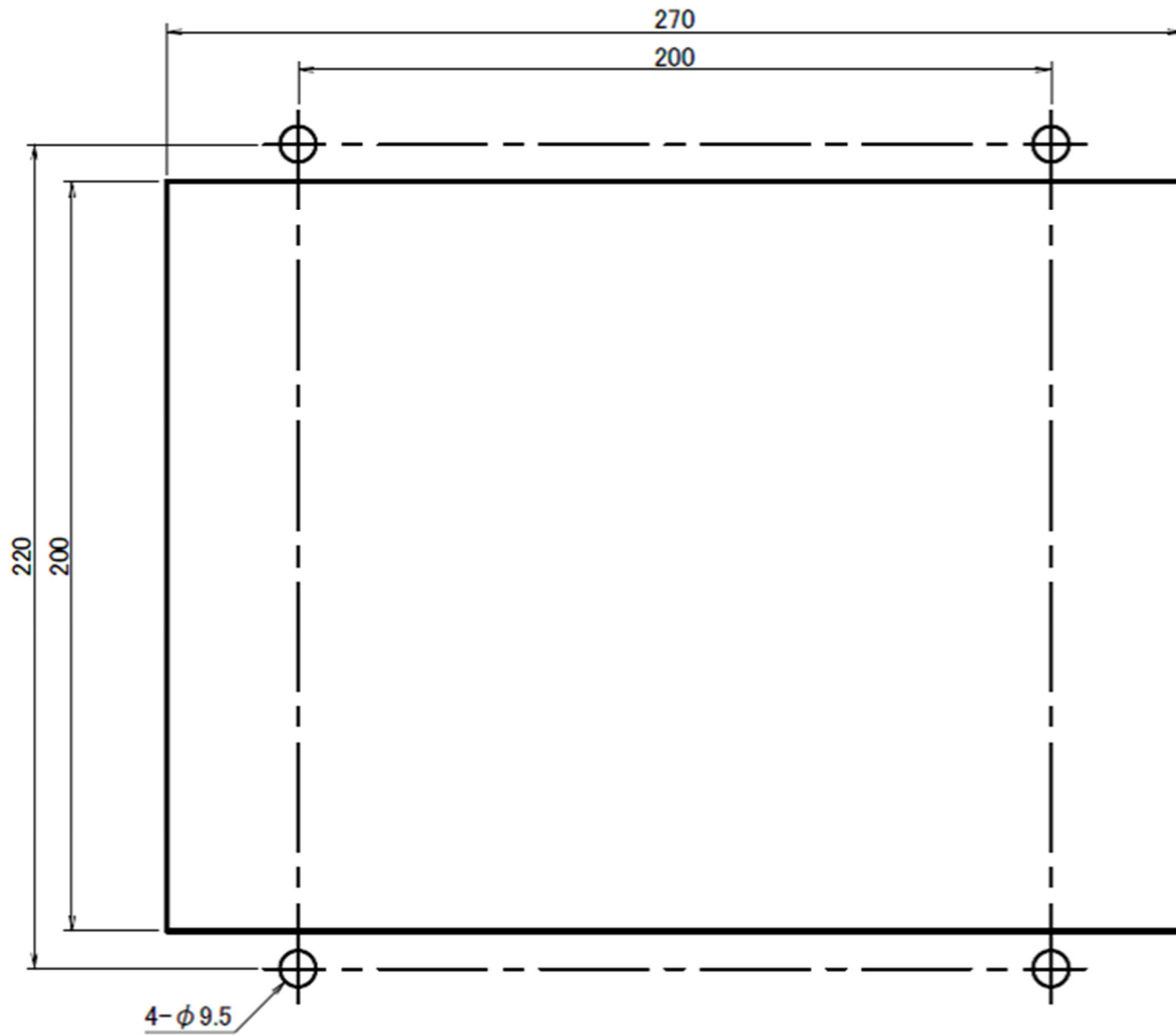
取付穴寸法図
