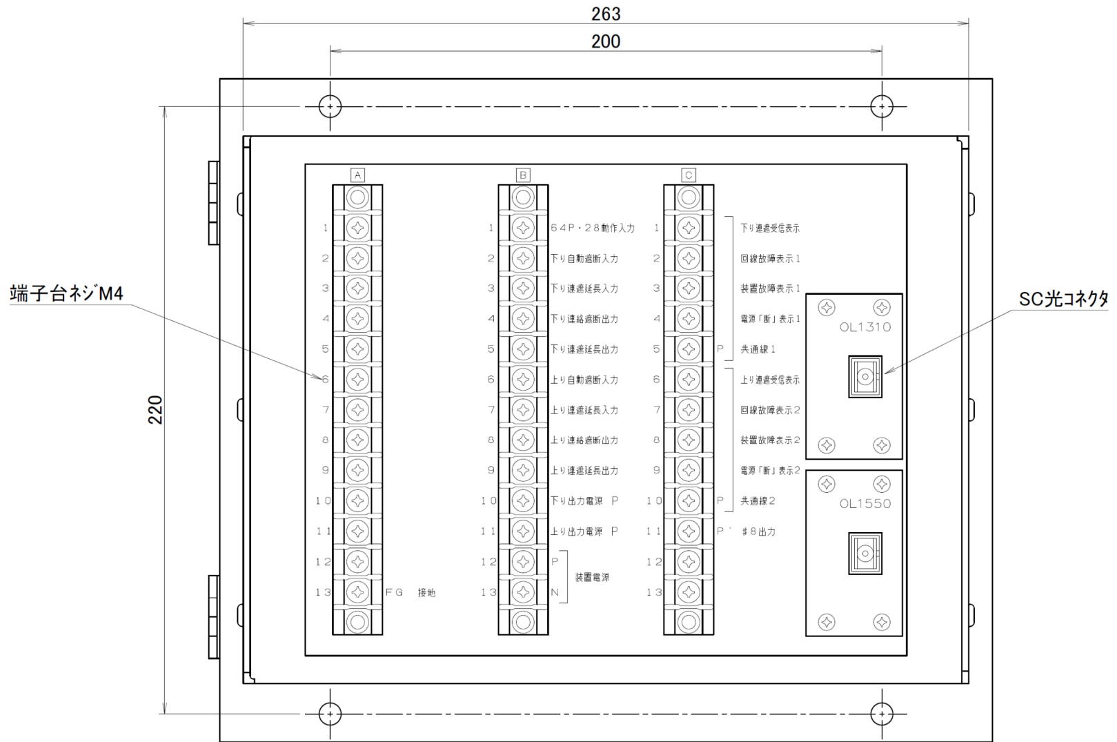
外部接続端子図
