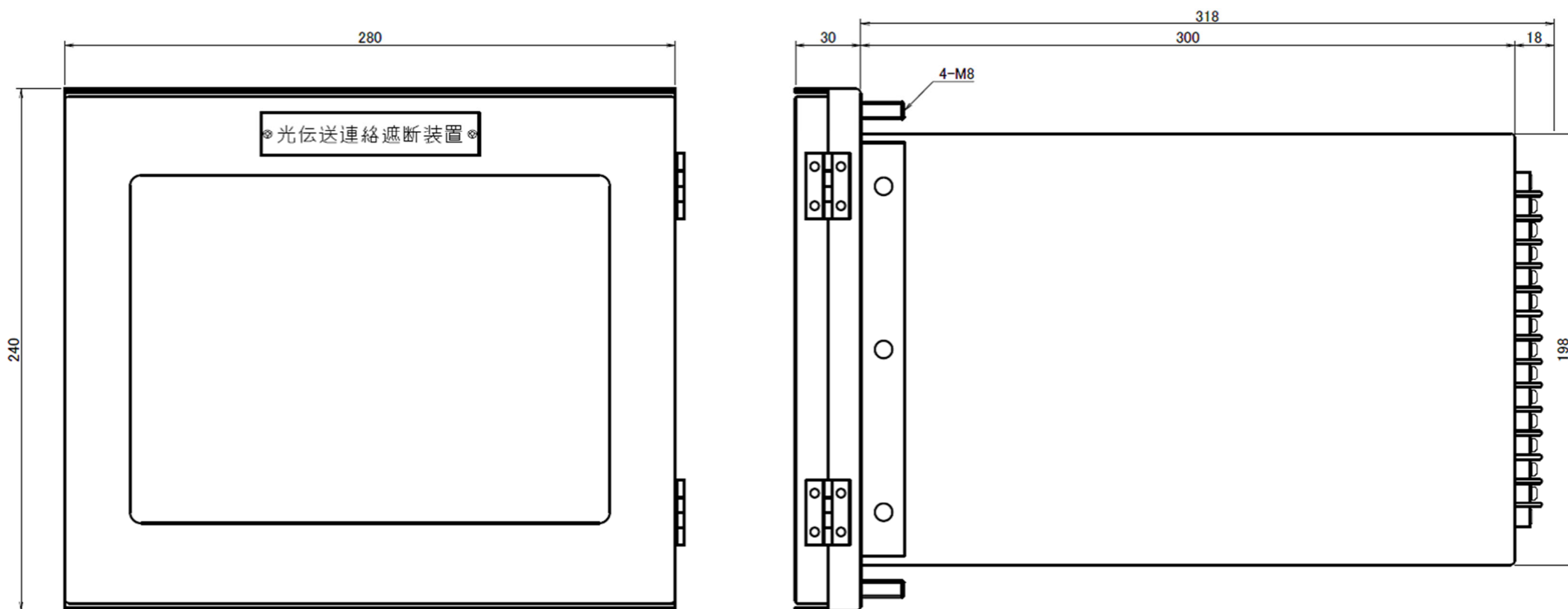
外形寸法図
