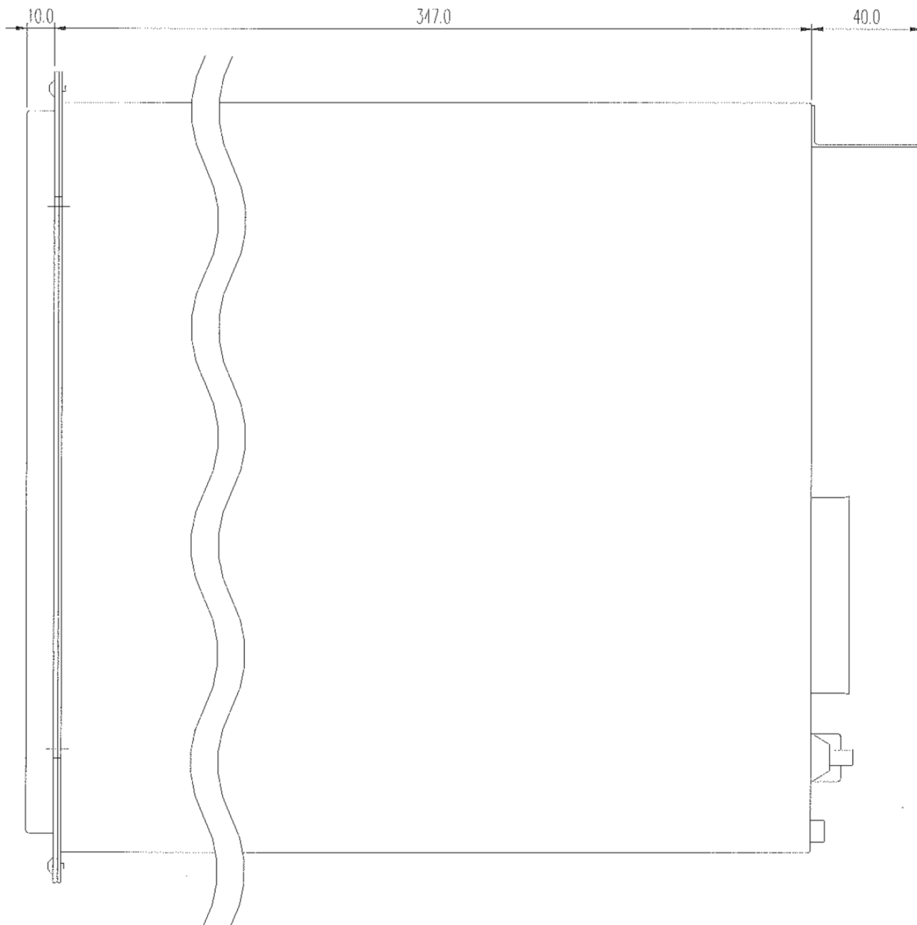
外觀図（側面）
